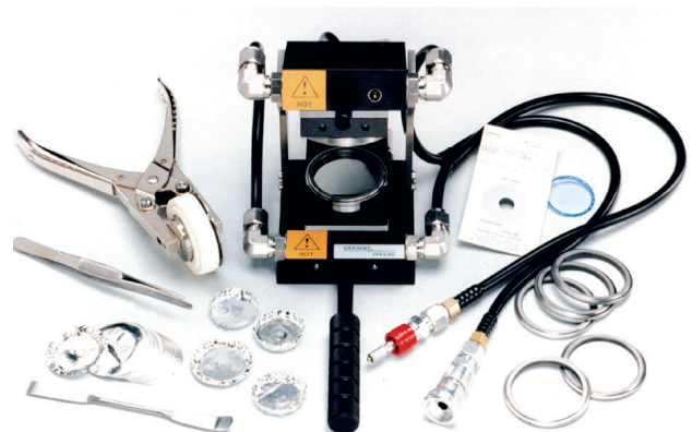
GS15800 高温定厚フィルム作製システム
